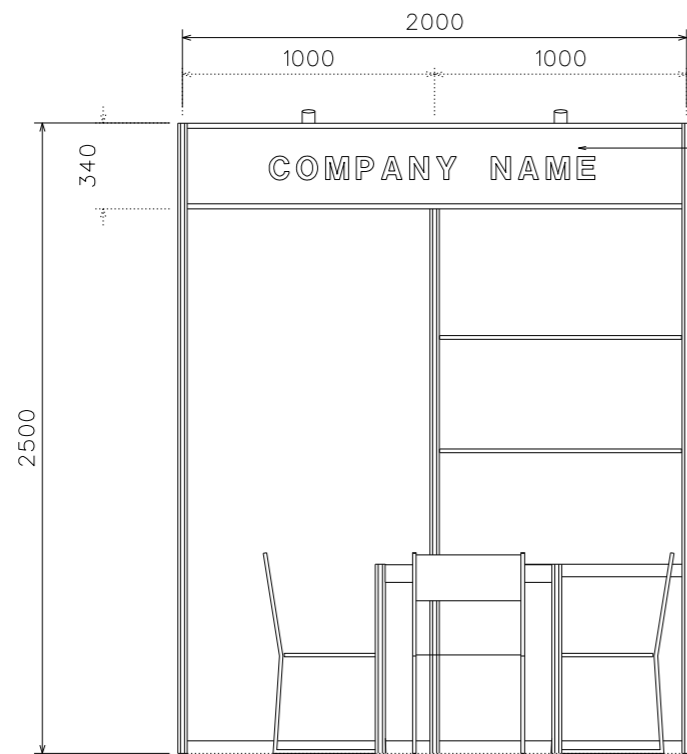
ELEVATION-A
