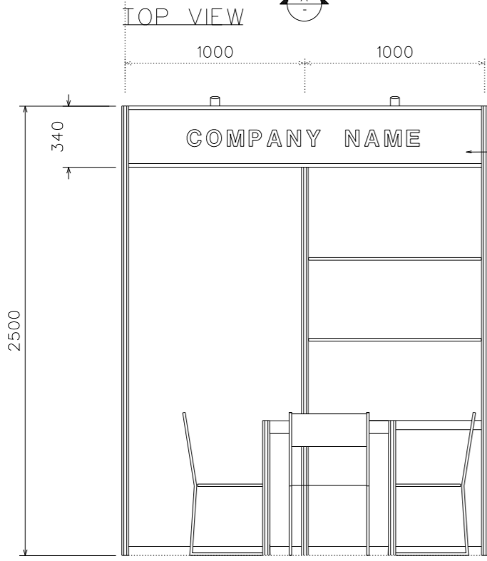
ELEVATION-A
