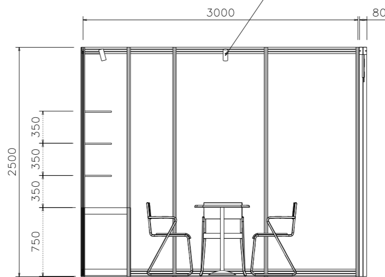
SECTION-A
