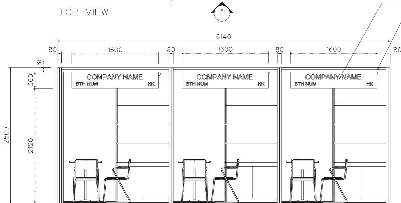
ELEVATION-A
