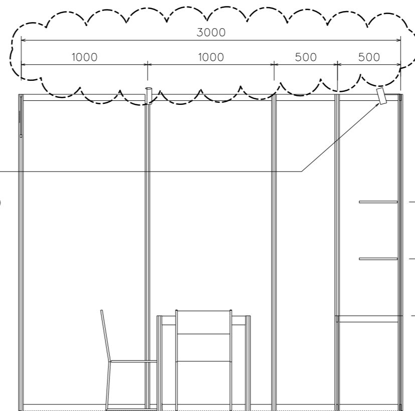
SECTION-A
